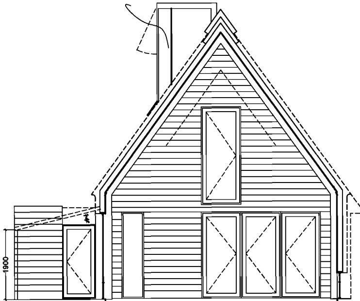
FACADE SYD
